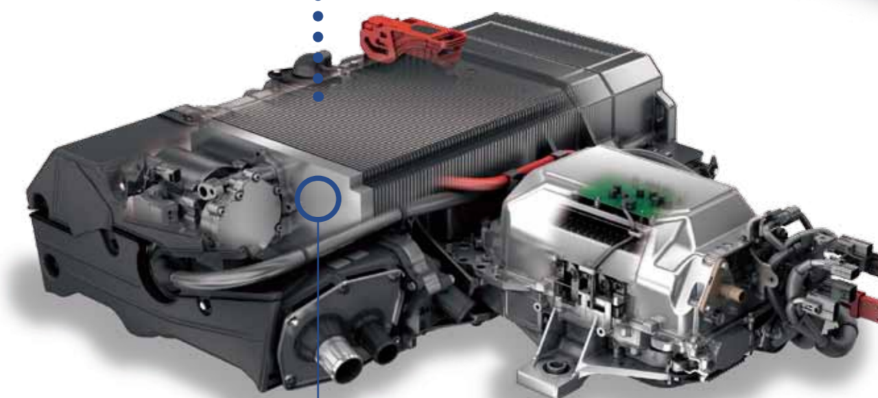
FCスタック部品 FC Stack Components
