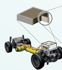
燃料電池FC セパレーター
